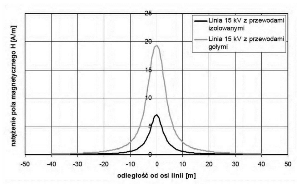
Ryc. 26. Rozkłady pola magnetycznego w otoczeniu linii napowietrznych średniego napięcia z przewodami izolowanymi i gołymi wyznaczone w miejscu największego zwisu przewodów przy minimalnej dopuszczalnej wysokości zawieszenia przewodów nad ziemią h=5 m (prąd linii I=475 A). Źródło: Jaworski M., Wróblewski Z. „Pole elektromagnetyczne w otoczeniu napowietrznych linii elektroenergetycznych”
